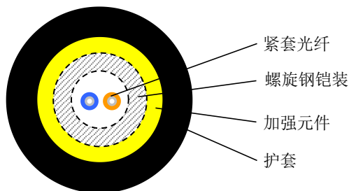
双芯圆形基站光缆IV型
